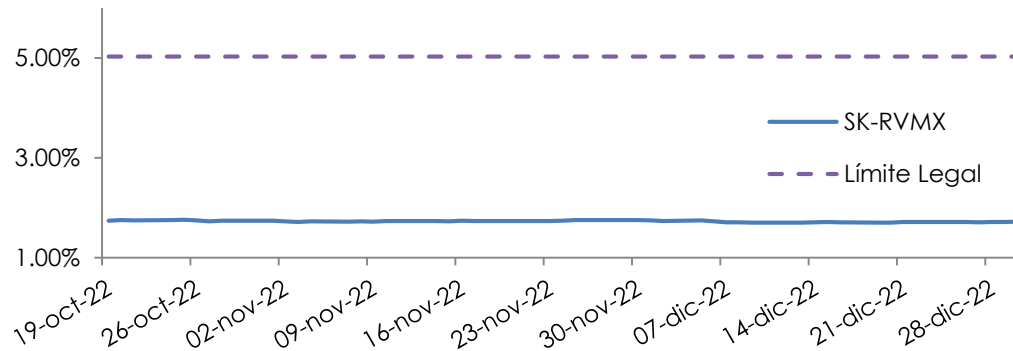
VaR SK-RVMX
