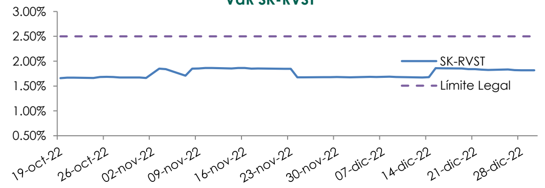
VaR SK-RVST
