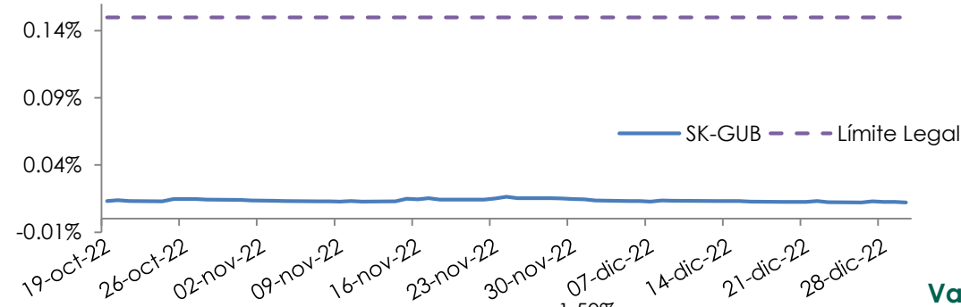
VaR SK-GUB
